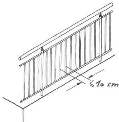
Figure 13 Géométrie des garde-corps, entraxe entre barreaux verticaux
